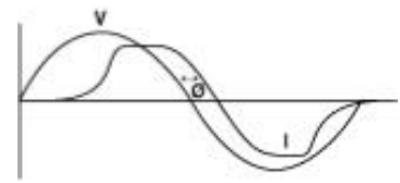
Figur 3: En icke-linjär strömkurva.
