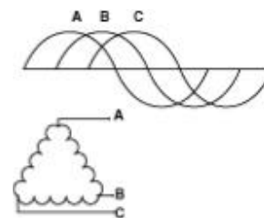
Figur 1: 3Ø- system med 3 ledare.
