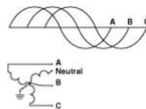
Figur 2: 3Ø- system med 4 ledare.
